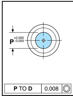
PESR TM P E E R L E S S E J E C T O R S H O U L D E R R O U N D
