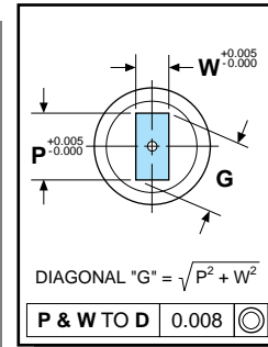
PESS TM P E E R L E S S E J E C T O R S H O U L D E R S Q U A R E / R E C T A N G U L A R
